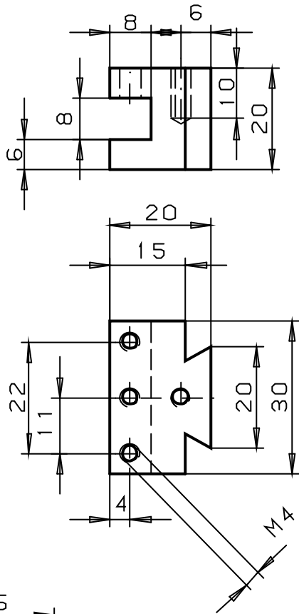
Stahlhalter
